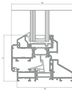
Querschnitt durch ein Fenster STEEL LOOK
