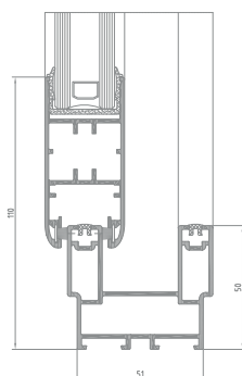
Slide Cold, Querschnitt eines 2-bahnigen Blendrahmens
