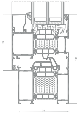
Querschnitt durch ein Fenster SP i+
