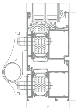
Querschnitt durch eine Tür IP 800 i+
