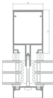
Querschnitt durch den Pfosten MC Passive +
