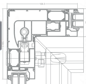
Querschnitt durch einen beweglichen Eckposten UG - Option mit Ecklösung
