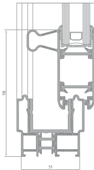
Querschnitt durch eine Tür SL+
