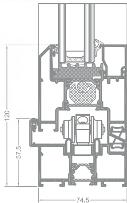
Querschnitt durch die Schwelle am Rahmen (nach innen öffnende Option) - Panorama i+
