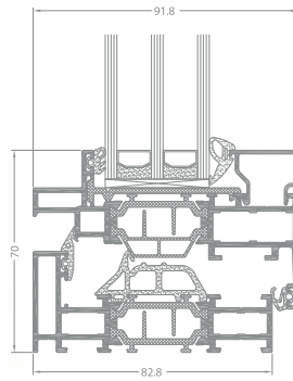
Querschnitt durch ein Fenster ML DESIGN
