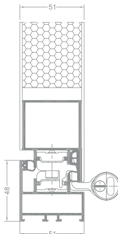
Querschnitt durch eine Paneeltür - Scharnierseite
