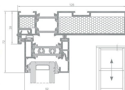
Außenflügel mit horizontalem Rahmen oben
