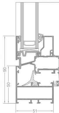
Querschnitt durch ein Fenster
