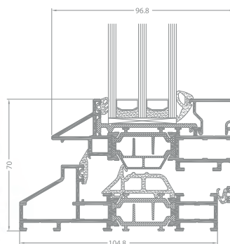
Querschnitt durch ein Fenster ML STEEL
