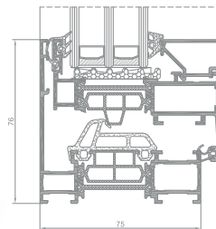
Querschnitt durch ein Fenster SP SU i
